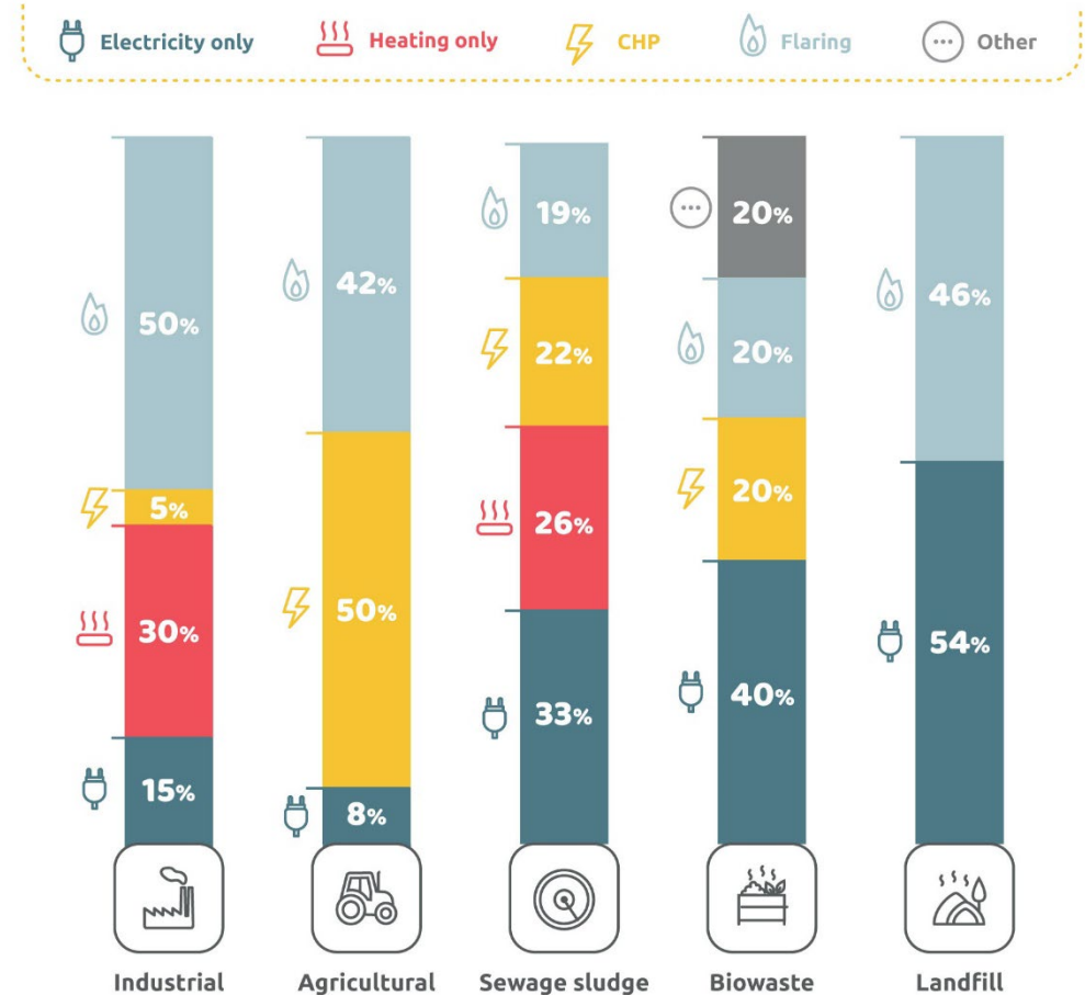
Biogas utilisation
